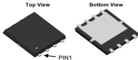
PDFN5X6-8L
